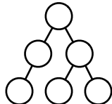
Tree(cache)
