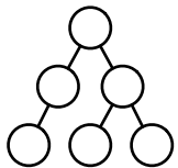
Tree(cache)
