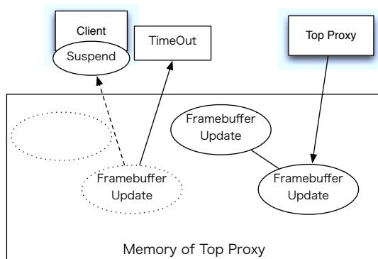
図 4 Timeout が代わりにデータを取得する
