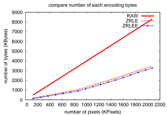
図 5 RAW, ZRLE, ZRLEE による 1 画面 (1920*1080) 描画にかかるデータ量。x 軸はピクセル数、y 軸はピクセル描画に必要なバイト数を表している。
