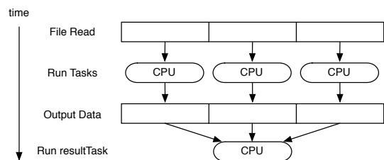
図 1: I/O を含む Task
