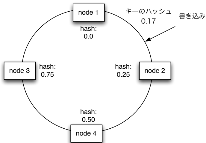
図 2.4: ConsistencyLevel QUORUM による書き込み
