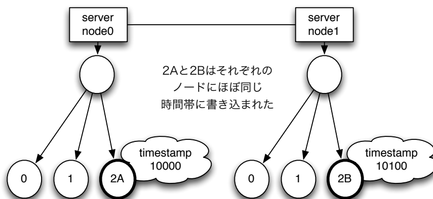
図 4.5: 他サーバノードの編集データ反映による整合性の崩れ 1
