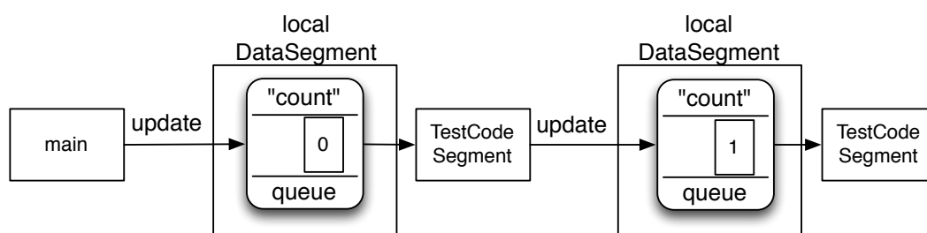
図 4.2: DataSegment と CodeSegment によるプログラムの例
