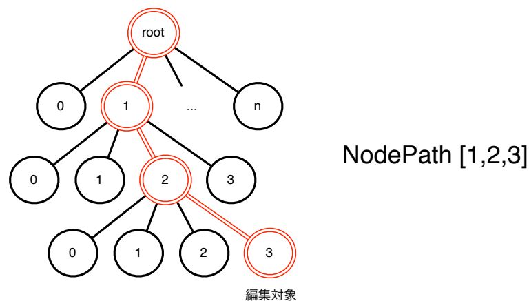
図 4.3: NodePath
