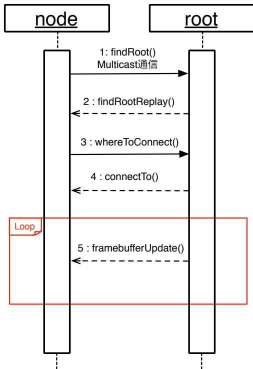
図 2.2: node 間で行われるメッセージ通信
