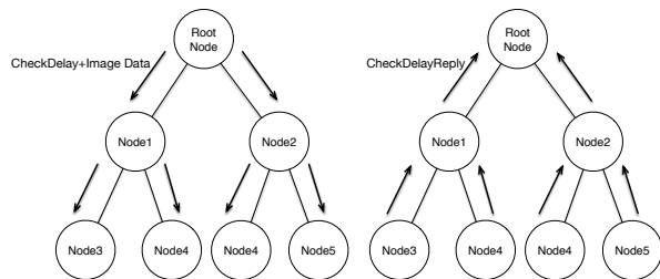
図 6 CHECK_DELAY, CHECK_DELAY_REPLY
