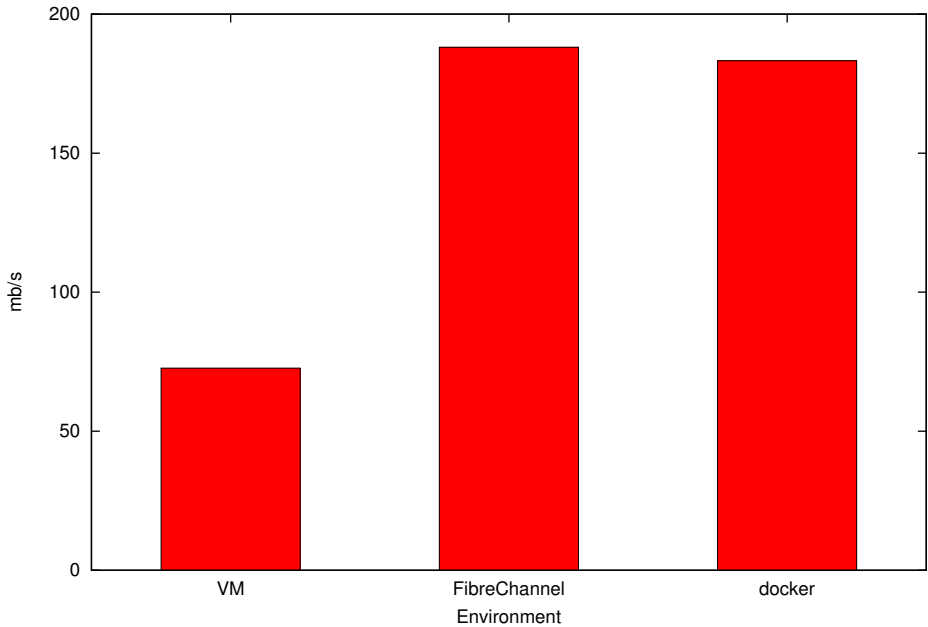
GFS2 benchmark
