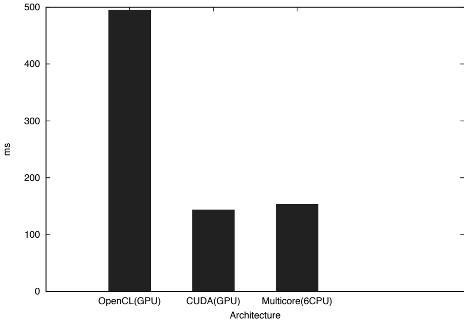
FFT Benchmark benchmark
