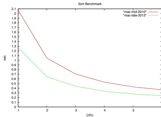
図 8.1: マルチコア CPU における Sort
