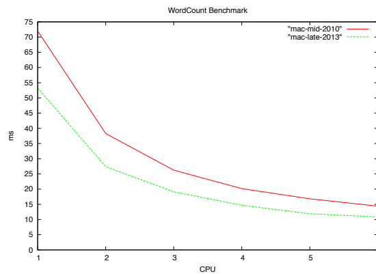
図 8.2: マルチコア CPU における WordCount
