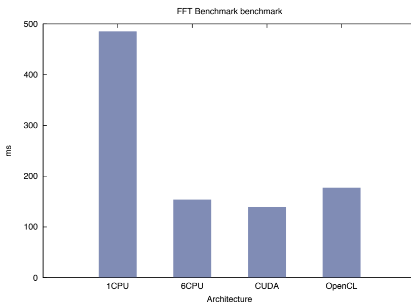
図 8.3: マルチコア CPU、OpenCL、CUDA における FFT
