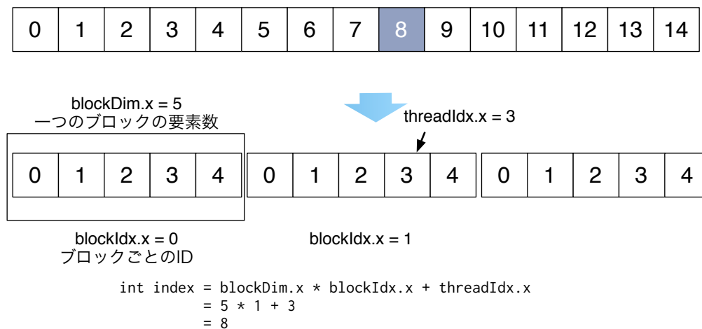
図 2.4: Calculate Index example
