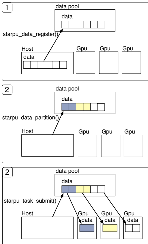
図 2.5: StarPU におけるデータ分割
