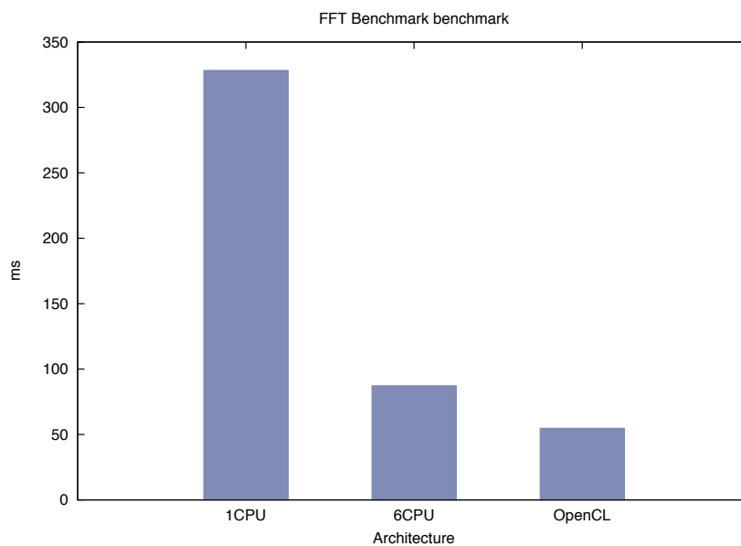
図 8.4: MacPro 2013 Late Model における FFT
