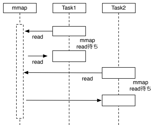
図 7.1: mmap の Model
