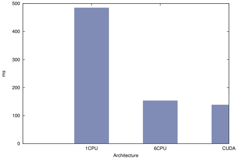
FFT Benchmark benchmark
