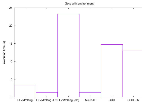
図 7.1: Mac OS X での Micro-C, GCC, LLVM/clang の実行速度比較グラフ
