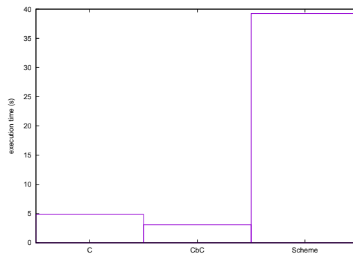
図 7.2: Mac OS X での C, CbC, Scheme の実行速度比較グラフ
