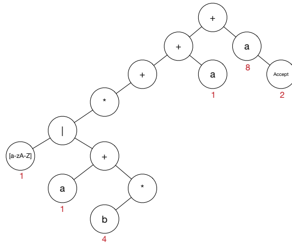
図 4.17: 与えられた正規表現をオートマトンに変換し、それに基づいて正規表現木に状態を割り振る
