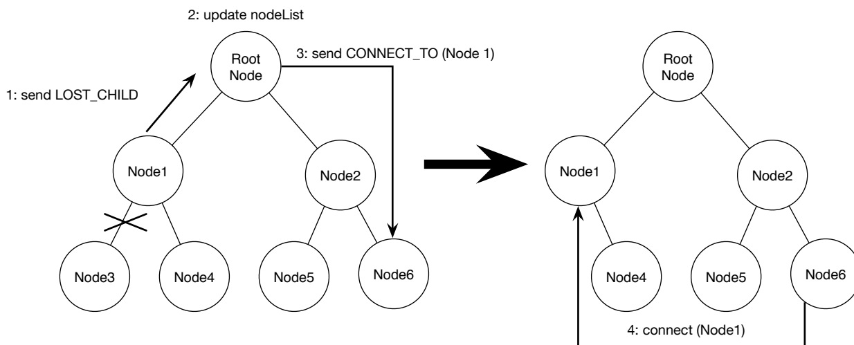
図 2.6: LOST_CHILD を検知・再接続
