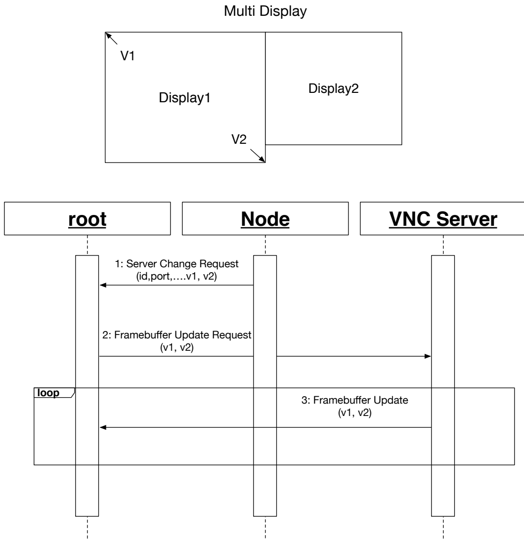
図 4.1: マルチディスプレイへの対応
