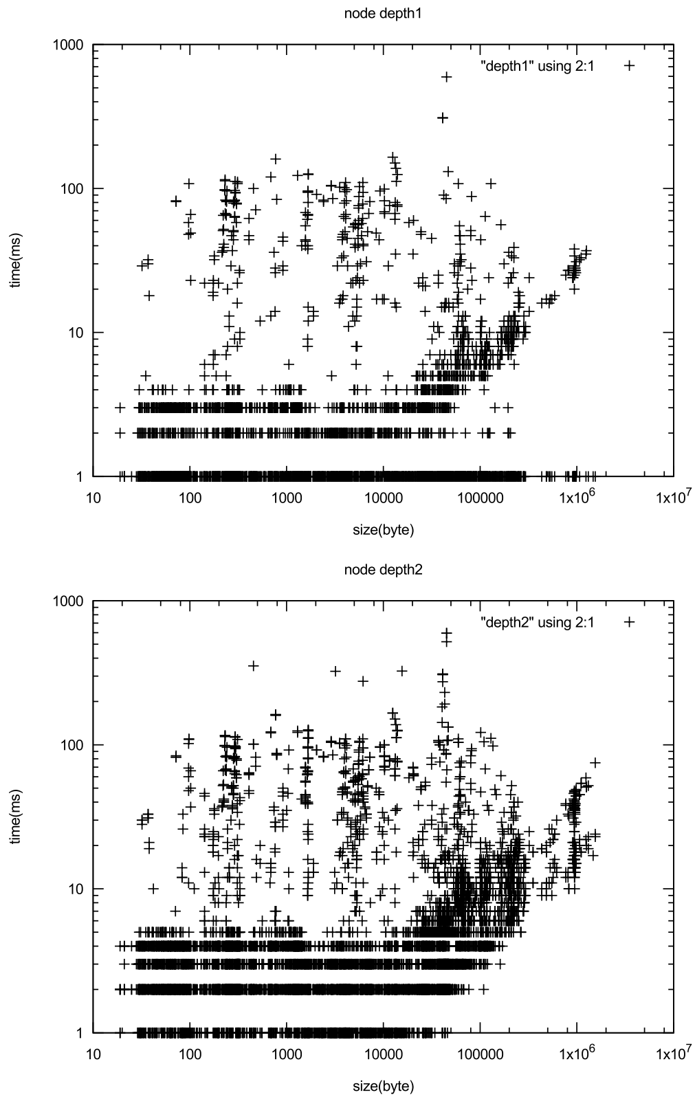
図 5.1: 深さ 1,2 のデータサイズと遅延の関係
