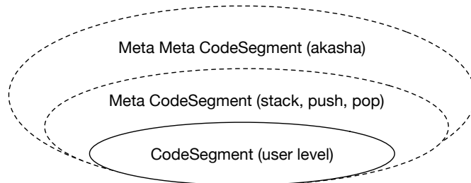
図 3.3: akasha とメタの階層構造
