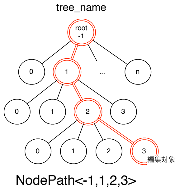
図 3.4: NodePath
