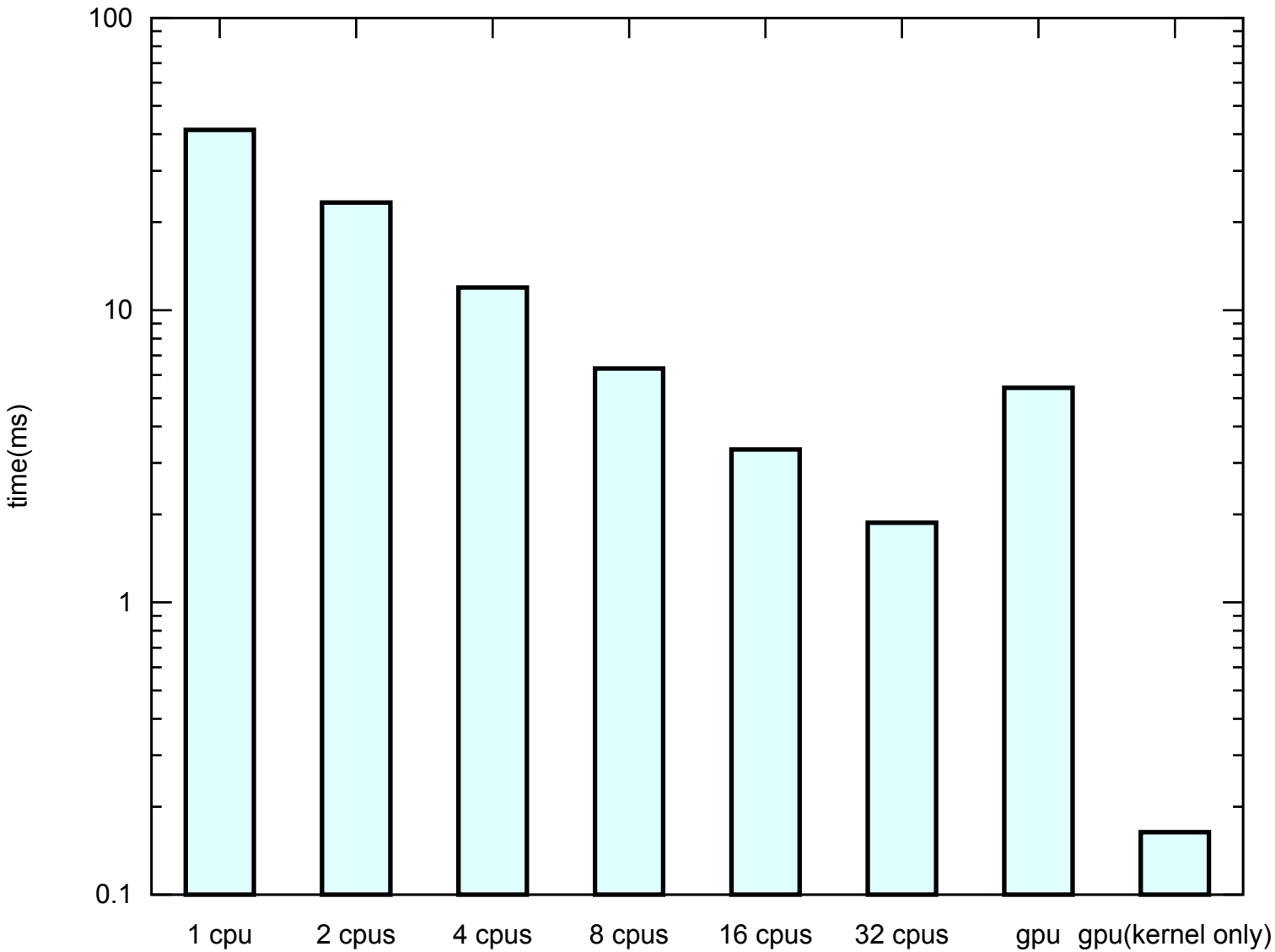
bitonicSort benchmark
