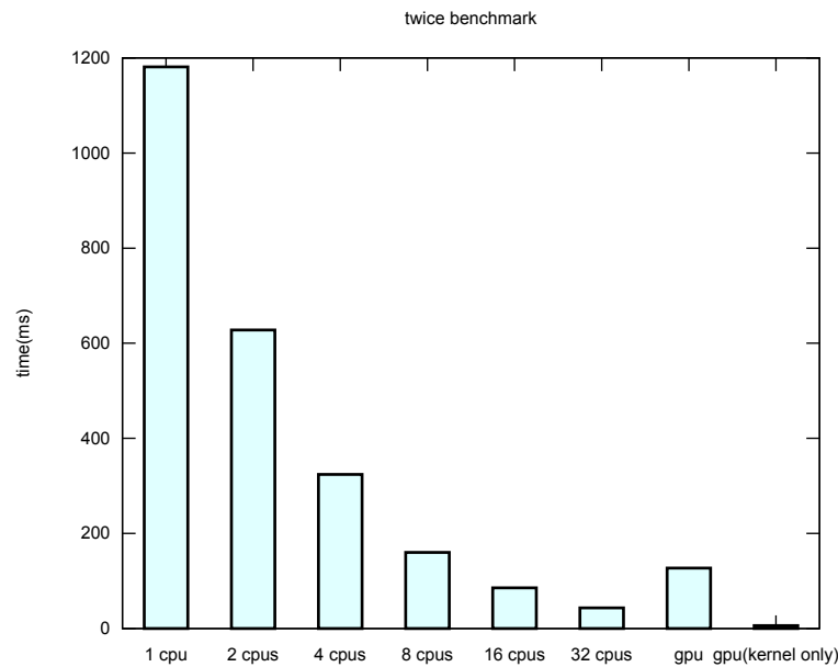
図 6.1: 2^{27} のデータに対する Twice
