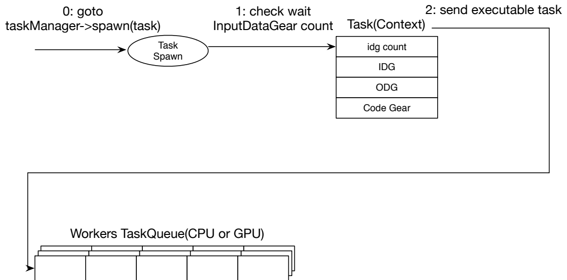
図 4.1: Worker への Task 送信
