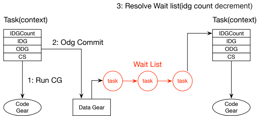
図 4.6: 依存関係の解決処理
