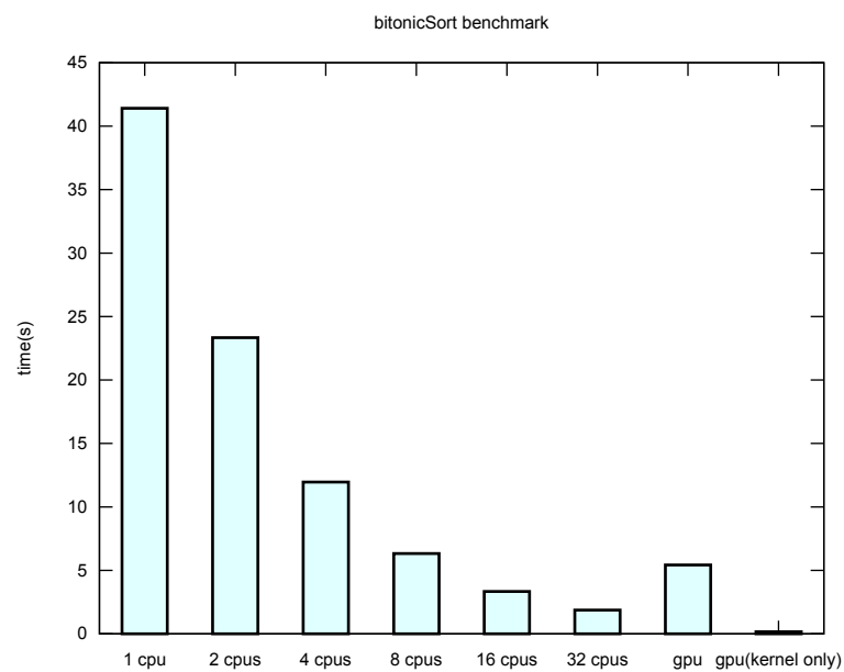
図 6.3: 2^{24} のデータに対する BitonicSort
