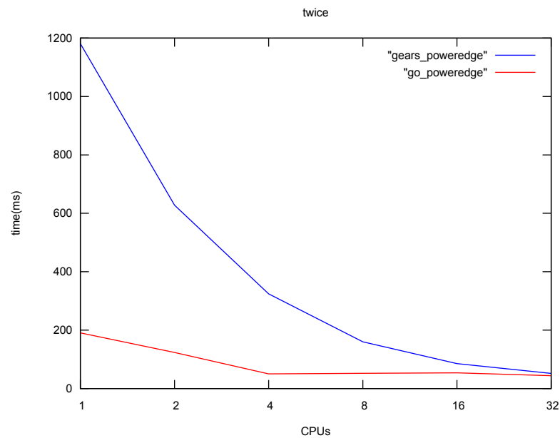
図 6.5: vs Go
