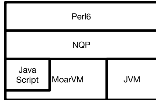
図 1: Rakudo の構成
