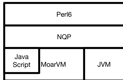
図 1: Rakudo の構成
