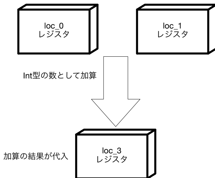
図 4.5: add_i 命令
