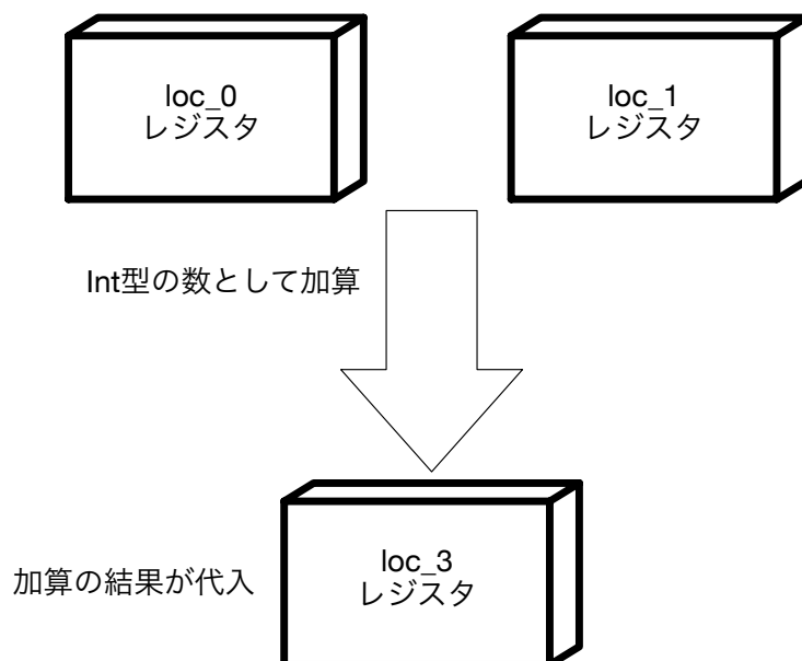
図 4.5: add_i 命令
