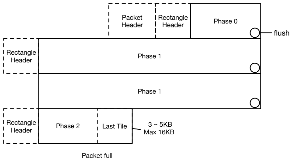
図 3.4: Rectangle と Packet の構成
