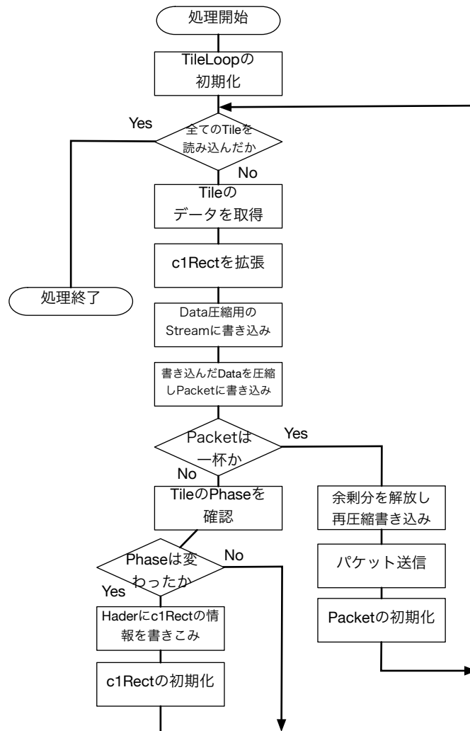
図 3.3: TileLoop のフローチャート
