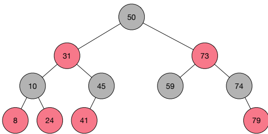
Figure 2: RedBlackTree の一例
