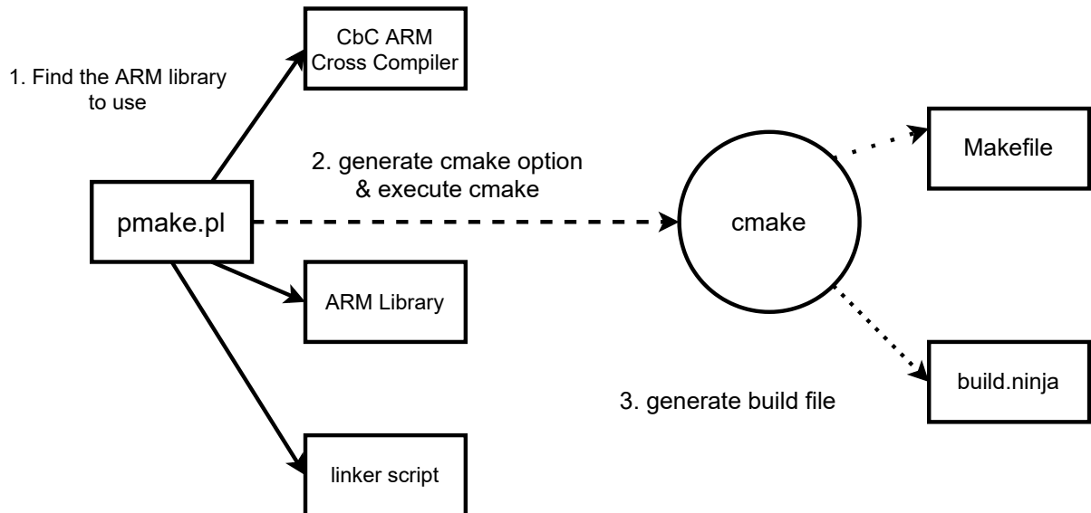
図 3.1: pmake.pl の処理フロー
