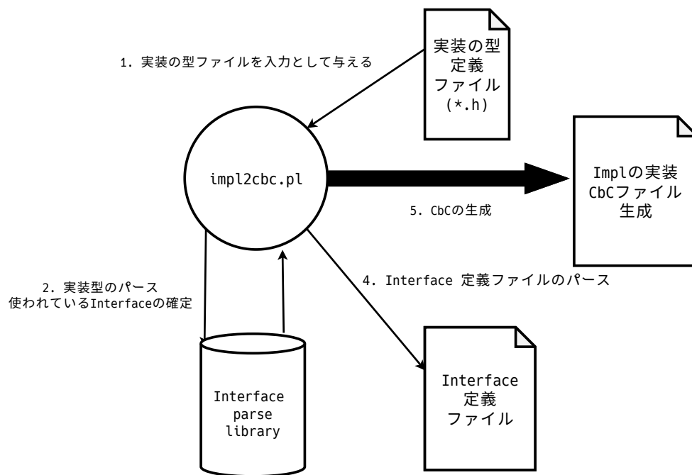
図 4.1: impl2cbc の処理の流れ
