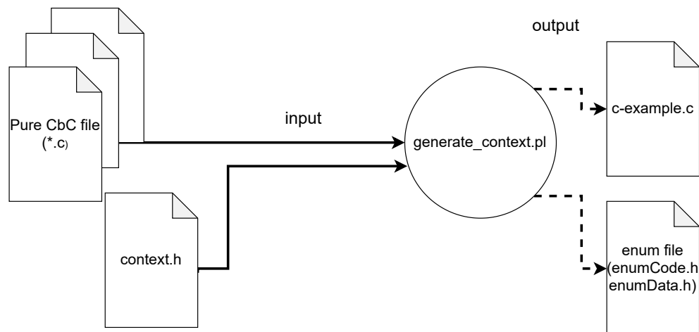
図 3.3: generate_context.pl を使ったファイル生成
