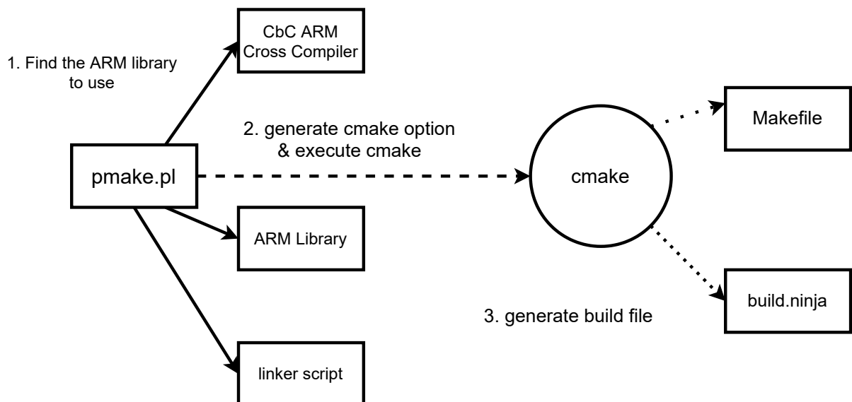
図 3.4: pmake.pl の処理フロー
