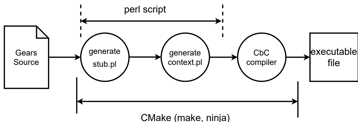
図 3.1: GearsOS のビルドフロー
