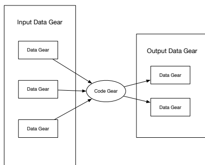
図 1: CodeGear と DataGear
